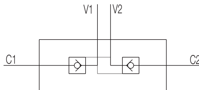
Hydraulisch Schema / Schema Hydraulique
